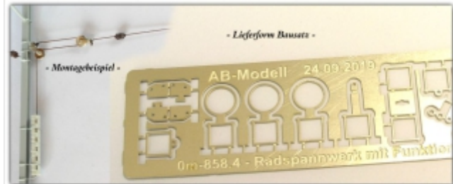
0m-858.4: Radspannwerk, ohne Anker, ohne Sockel, für 4mm-H-Profil, mit Funktionselement (Sommerfeldt)
