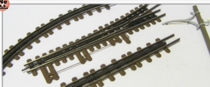
Ne-502.0: Riggenbach-Zahnstangenweichen/-gleise, 4,5 mm Oberleitungsausleger der SPB, Messingbausatz
