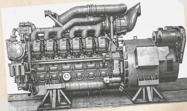
Motore FIAT A210.12 da 95,700 cm 3 con a destra l'alternatore calettato.
